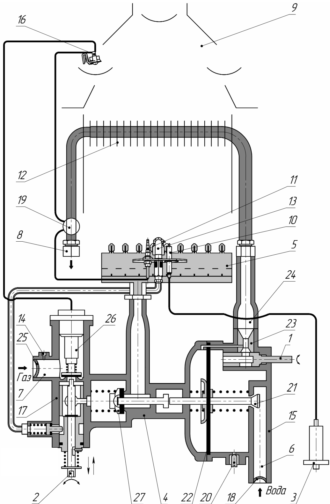
1 – регулятор расхода воды; 2 – регулятор расхода газа; 3 – устройство пьезорозжига; 4 – узел водогазовый; 5 – горелка; 6 – подвод холодной воды; 7 – подвод газа; 8 – отвод горячей воды; 9 – газоотводящее устройство; 10 – свеча розжига; 11 – термопара; 12 – теплообменник; 13 – запальная горелка; 14 – штуцер замера давления газа; 15 – узел водяной; 16 – термореле (датчик наличия тяги); 17 – узел газовый; 18 – фильтр водяной; 19 – термореле (датчик перегрева воды); 20 – пробка для слива воды; 21 – ограничитель расхода воды; 22 – мембрана; 23 – штуцер Вентури; 24 – выход воды к теплообменнику; 25 – фильтр газовый; 26 – электромагнитный клапан; 27 – клапан газовый.
