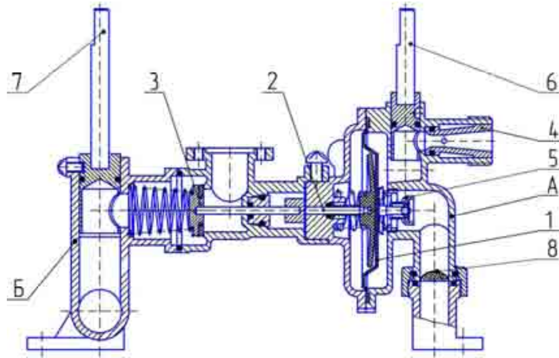
Рисунок 2 Блок водогазовый
